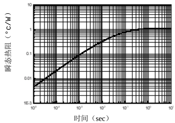
图四、热 响 应
