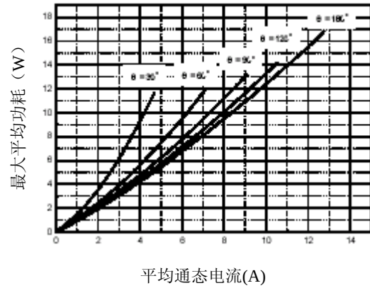
图八、功耗
