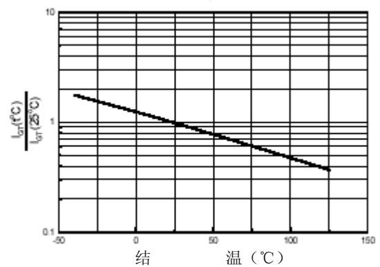
图六、典型门极触发电流----结温
