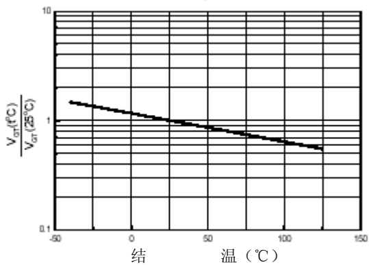
图五、典型门极触发电压----结温
